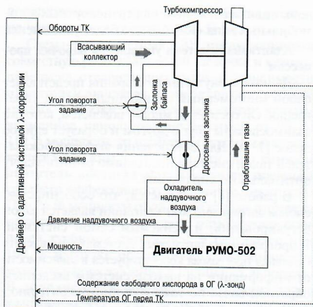
Рис. 7. Схема адаптивной системы управления газовым двигателем РУМО-502
