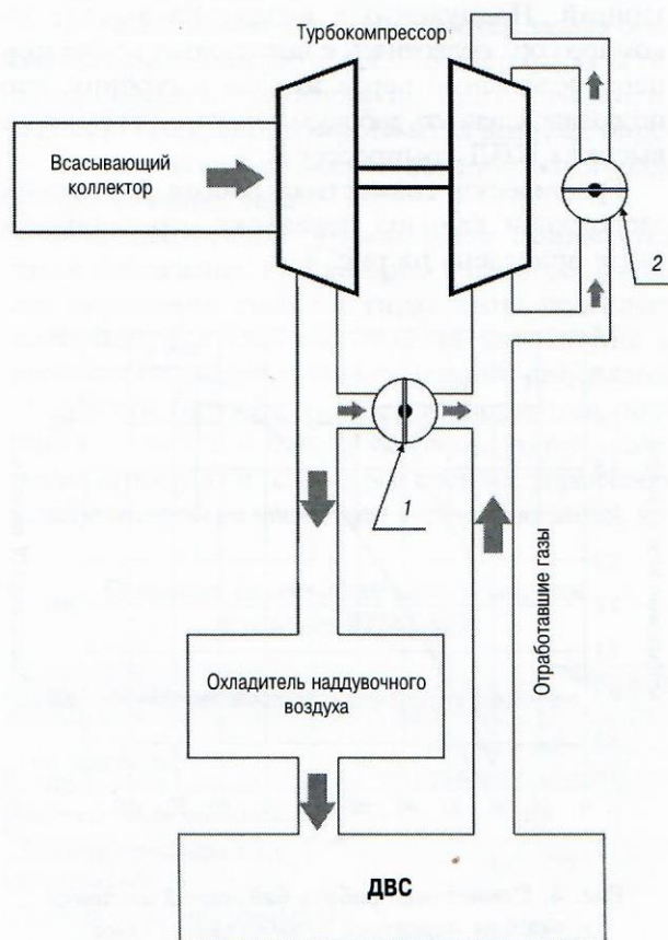
Рис. 3. Система управления воздухообеспечения цилиндров двигателя:
